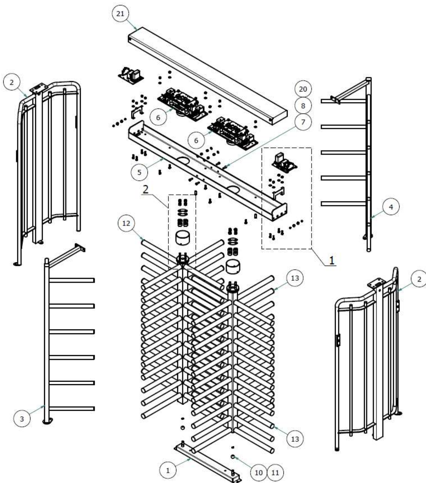
Abbildung 13: Montage des 3-arm Doppel-Drehkreuzes
