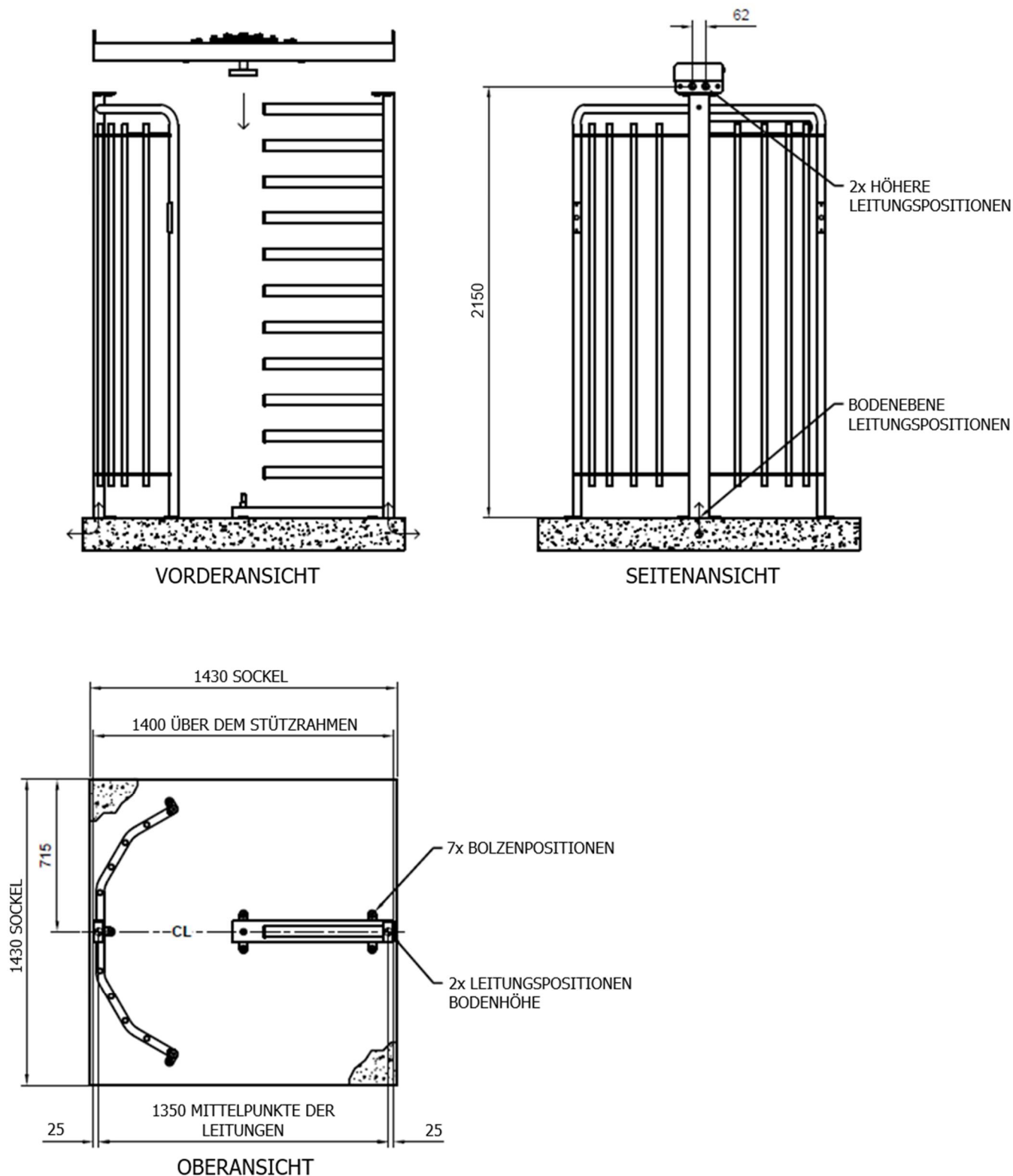
Abbildung 11: Einzel-Drehkreuze-Montage
