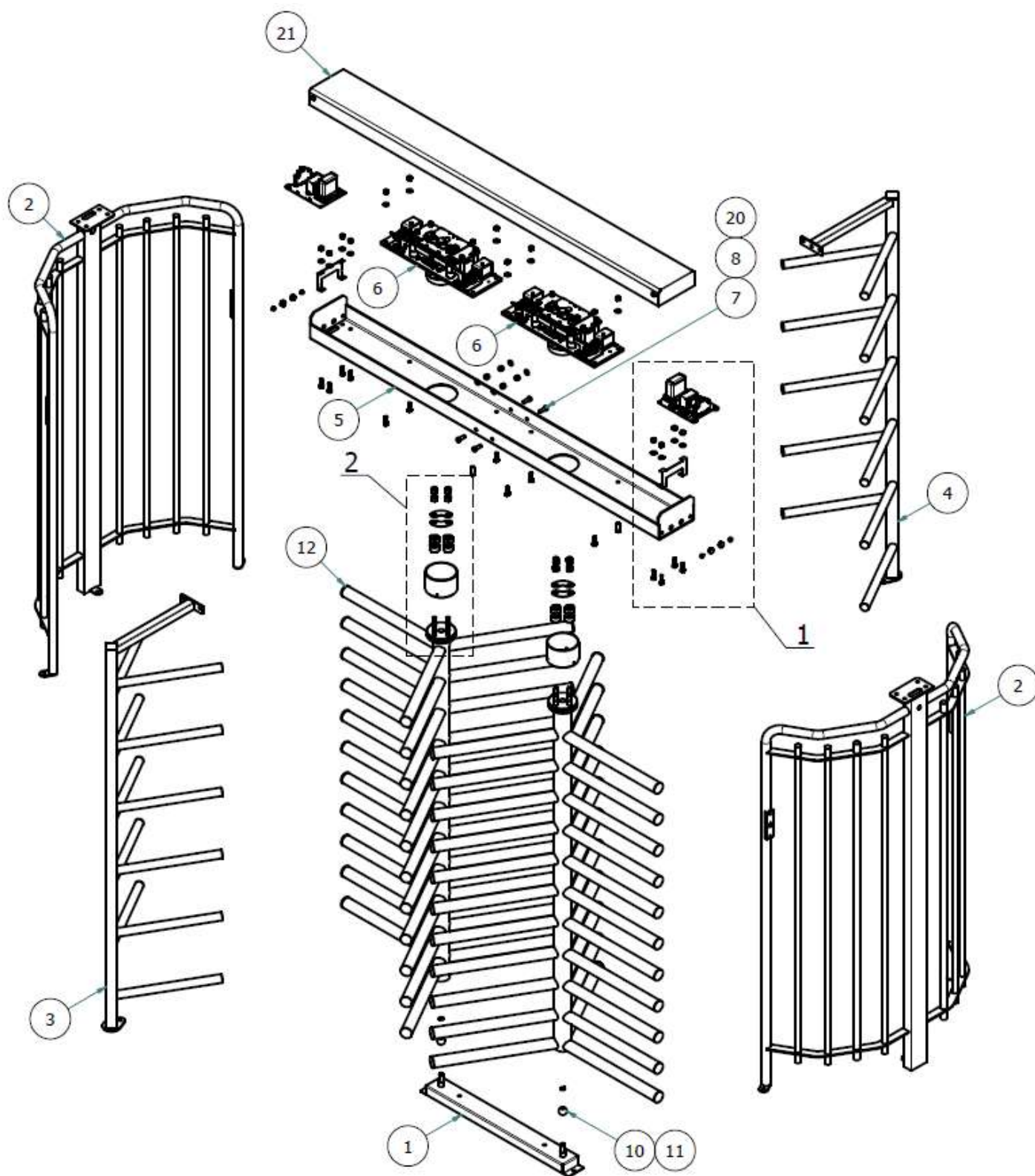
Abbildung 12: Montage des 3-arm Doppel-Drehkreuzes
