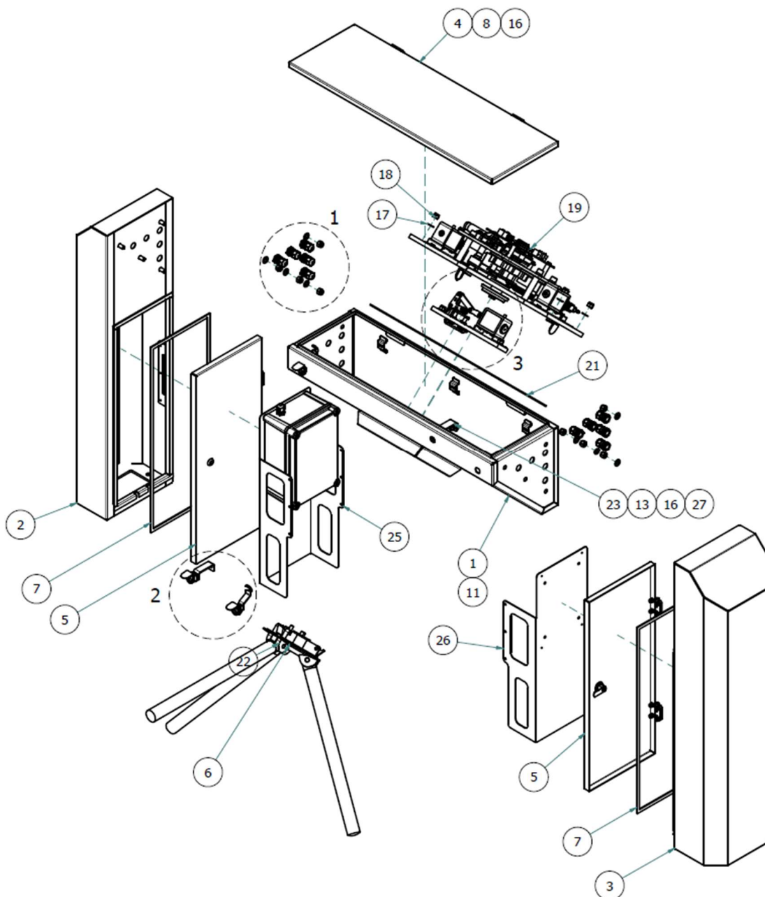
Abbildung 3: Explosionsansicht des Streamlines
