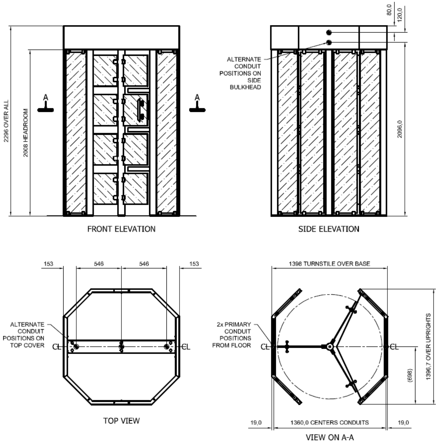
Abbildung 2: Eindrehkreuz-Rohre
